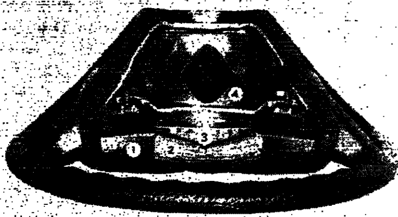
Versuche zeigen die Wirkung des Airbag (rechts). Sein System im Schnitt: Polsterplatte (1), Luftsack (2), Gasgenerator (3), der Prellkoppl (4).
